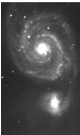
Galàxia M51, telescopi de 20 cm. Milions d'estrelles i immensos núvols de gas i pols dibuixen els braços espirals d'aquesta galàxia. Fotografia i imatges extretes del de l'observatori
